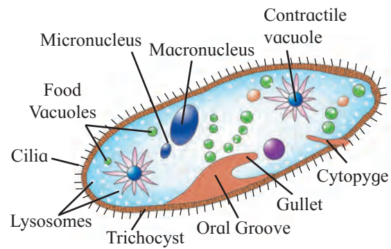
Fig. 2.8 Paramecium
