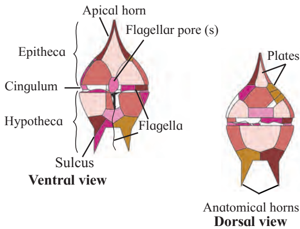
Fig. 2.6 Gonyaulax
