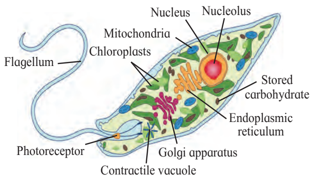
Fig. 2.7 Euglena
